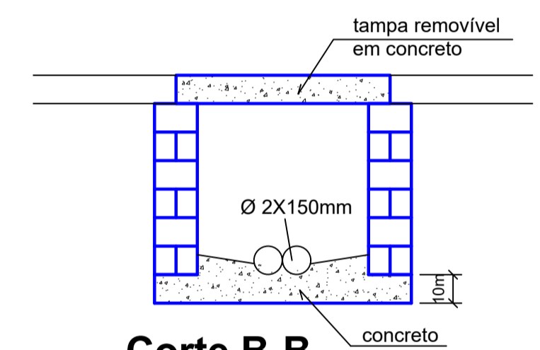
Corte B-B sem escala
