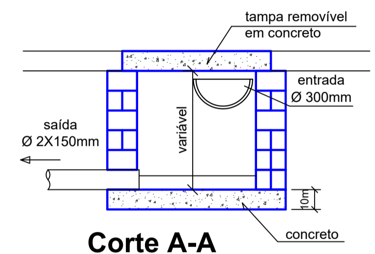
Vista Superior sem escala
