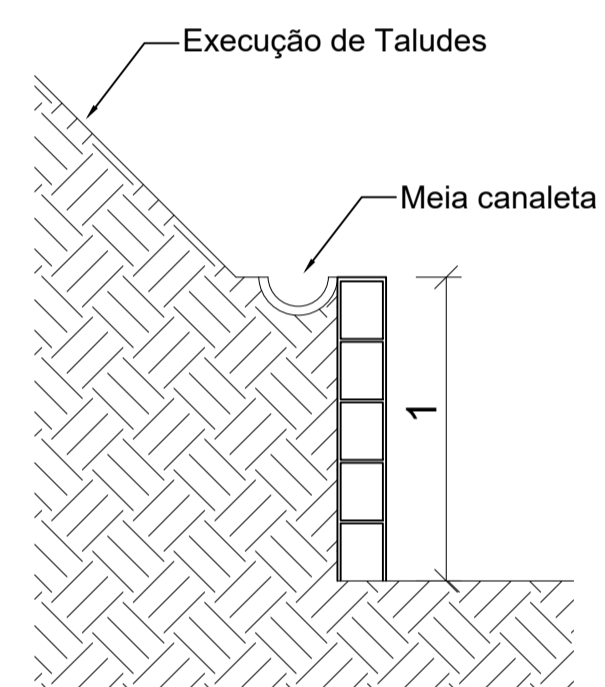
CORTE MURO Esc: 1/25
