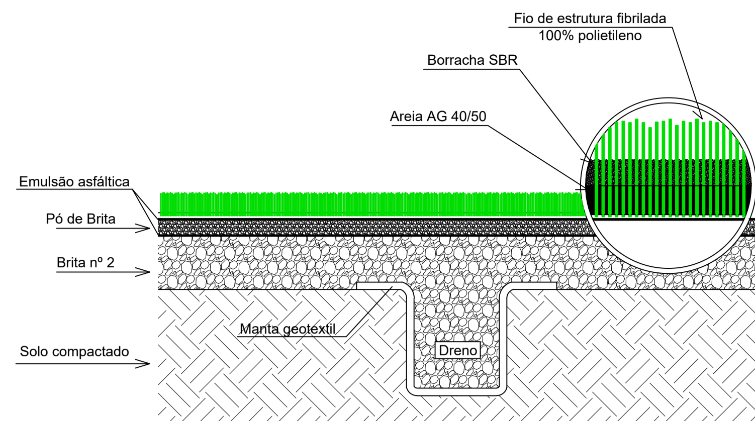
DETALHE GRAMA SINTETICA Sem escala
