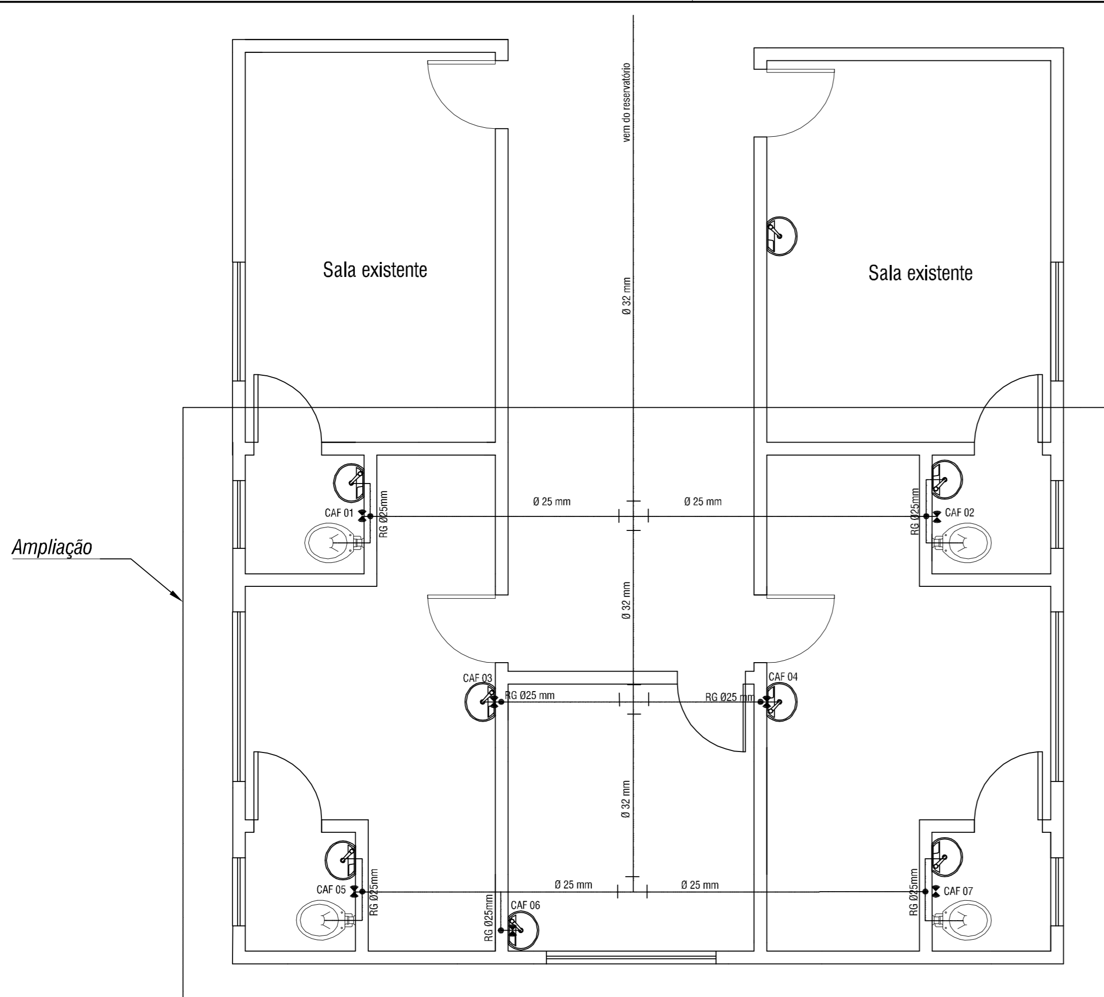
PROJETO HIDRÁULICO ESC - 1:50
