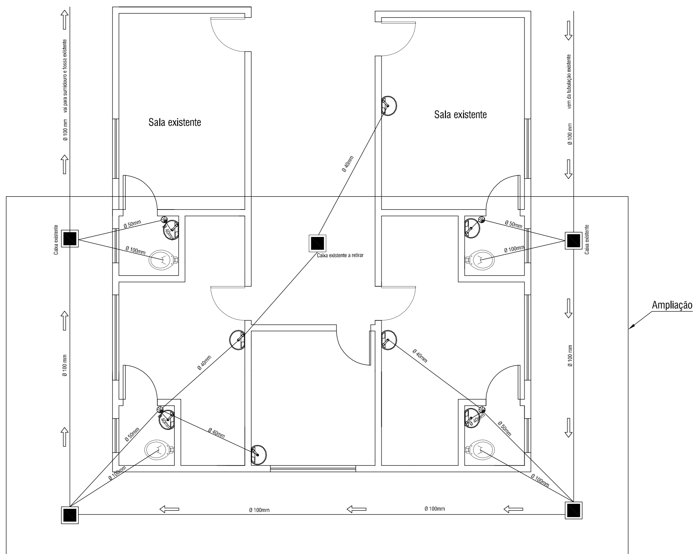
PROJETO SANITÁRIO ESC - 1:50
