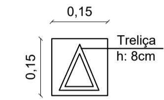
Pilares e vigas das platibandas
